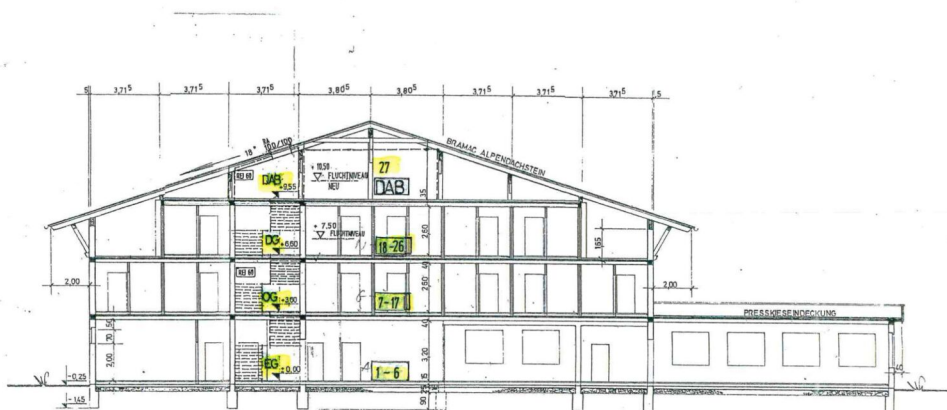
SCHNITT A-B
